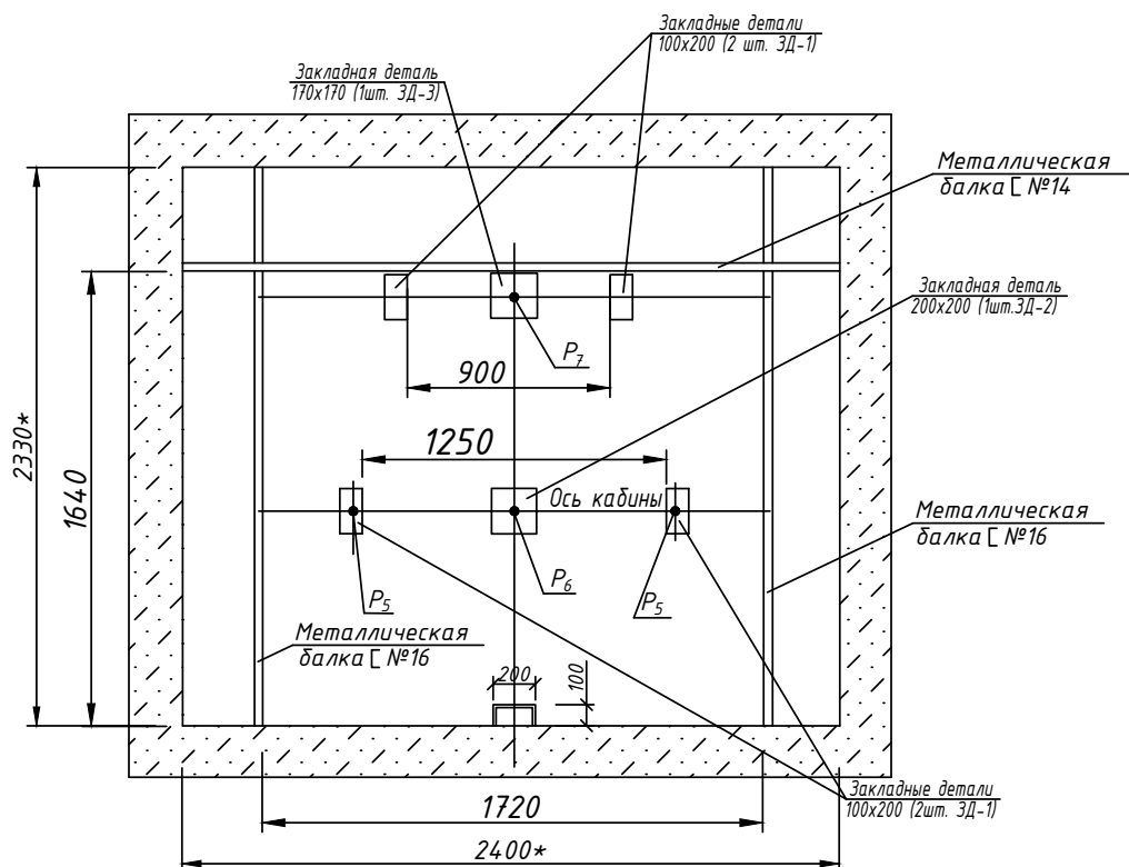
План прямка шахты (Б-Б)
