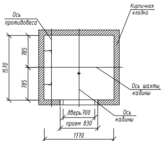
План шахты (А-А)
