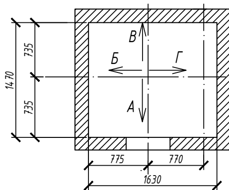
План шахты
